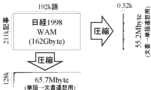
図 2. WAMの圧縮
