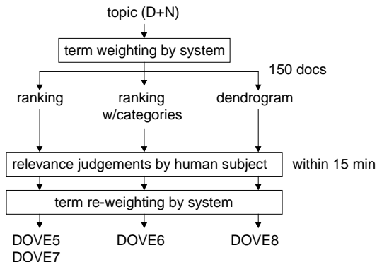
図 1: 対話的 run の概要
