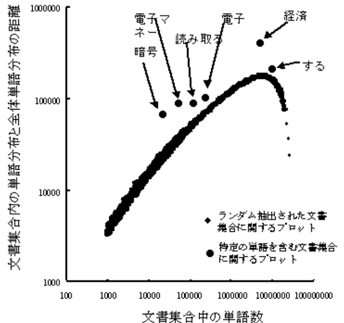
図 4. 文書集合中の単語の偏り
