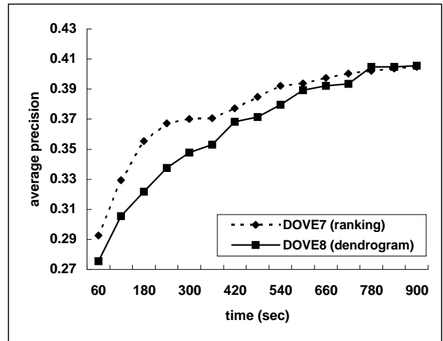
図 2: 平均精度の時間推移
